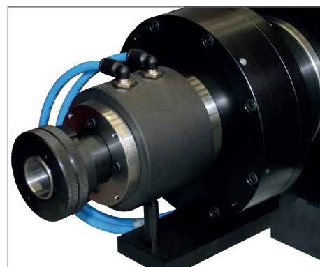
Serrage pneumatique Pneumatische Spannung Pneumatic clamping
